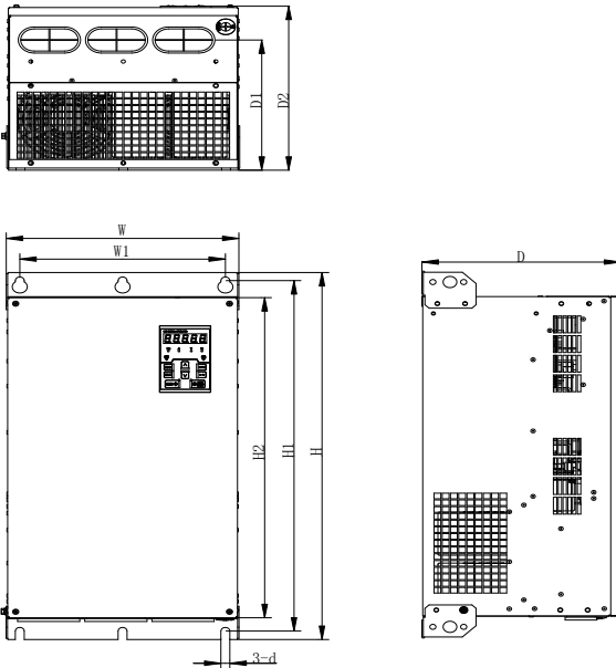
(b) 90kW~160kW 变频器外形
